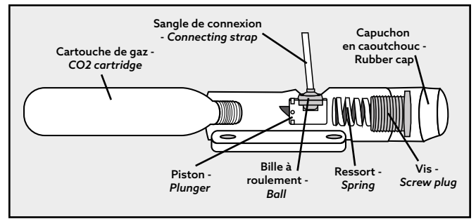
Structure du système - System structure
